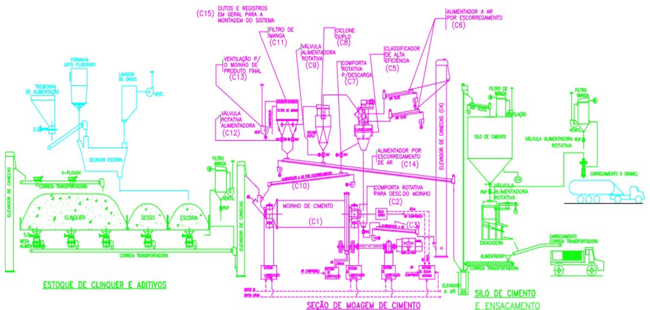
Figura 05: Fluxograma do processo produtivo – Etapa Final
