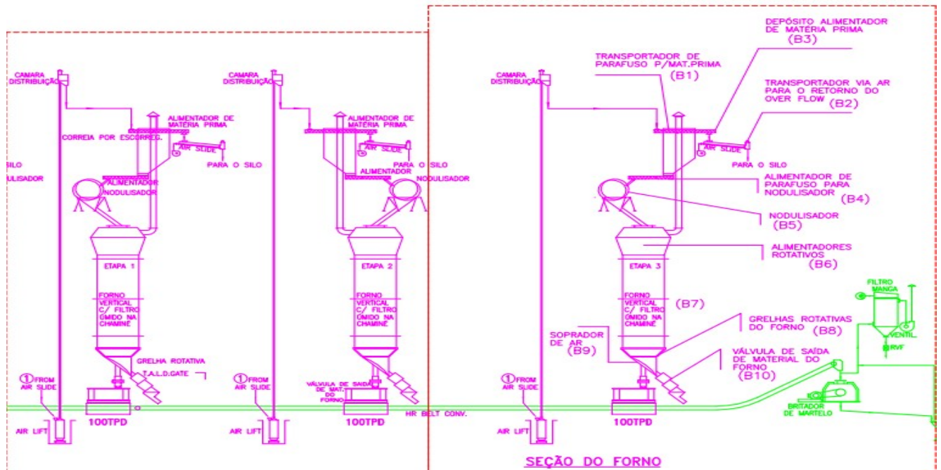
Figura 04: Fluxograma do processo produtivo – Etapas 01, 02 e 03
