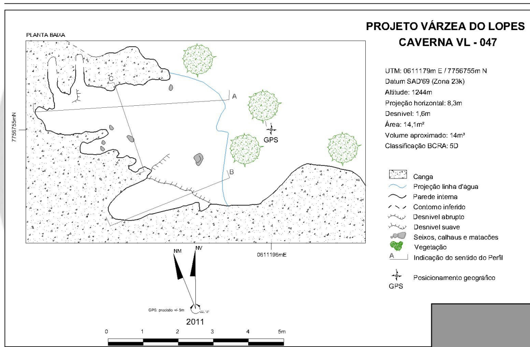
Figura 1: Planta baixa da Cavidade VL-47. Fonte: Estudos de redução de raio
